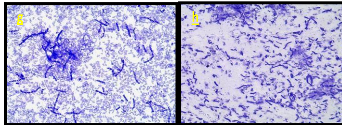
Bacillus insolitus
